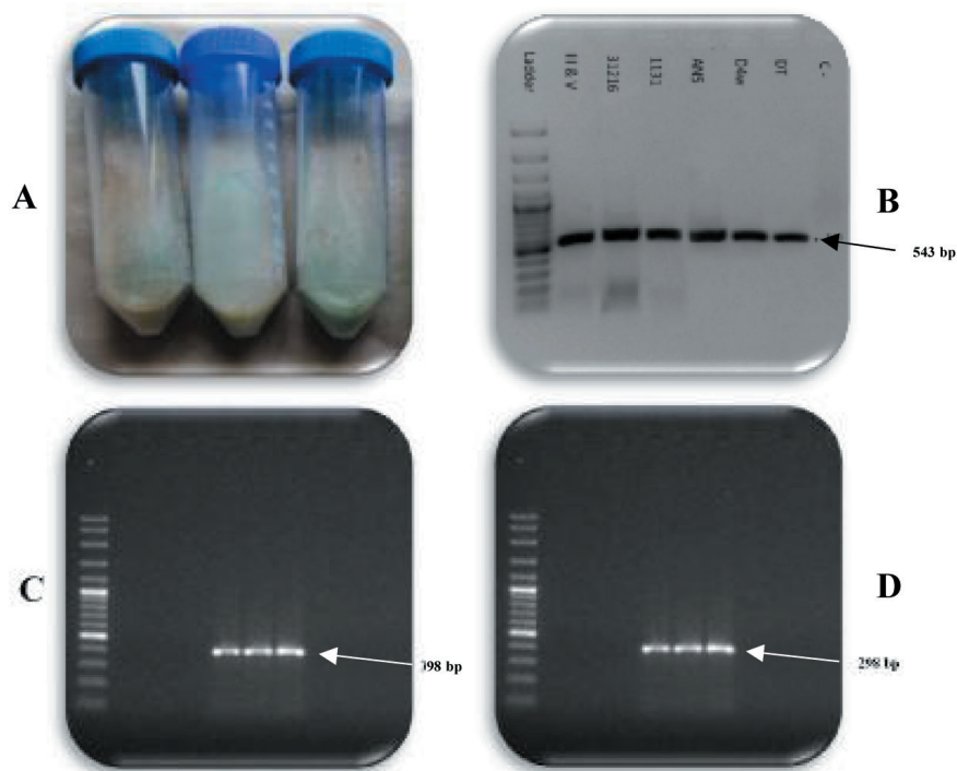
شکل ۱- A: رشد پرگنه های MAP در لوله کشت محتوی محیط کشت Herrold's egg yolk همراه با مایکوباکتین ز. B: تولید یک قطعه به طول ۵۴۳ bp در آزمایش PCR-rRNA ۱۶S توسط جدایه‌های MAP. C: تولید یک قطعه به طول ۳۹۸ bp در آزمایش PCR-IS۹۰۰-۹۱/P۹۰ توسط جدایه‌های MAP. D: تولید یک قطعه به طول ۲۹۸ bp در آزمایش PCR-IS۹۰۰-AV۱/AV۲ توسط جدایه‌های MAP. چیدمان چاهک‌ها در C و D به ترتیب راست به چپ چاهک شماره ۱ سبزی مارکر، چاهک شماره ۲ Blank، چاهک شماره ۳ کنترل منفی، چاهک شماره ۴ سویه مایکوباکتریوم اویوم زیر گونه اویوم و چاهک شماره ۵ تا ۷ سویه‌های واکسن پاراتوبرکلوز MAP III&V و MAP ۲۱۶F و جدایه ۲۴۸۸۳.
